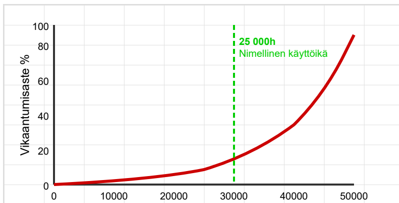
Käyttöikäkaavio - 25 000 tunnin nimellinen käyttöikä
