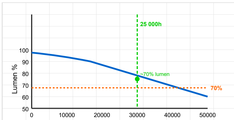
Lumenin ylläpitokaavio - Valovirran lasku ajan myötä
