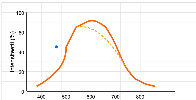
MAS LEDspot VLE D 9.5-75W 930 PAR30S 25D - 3000K lämmin valkoinen spektri
