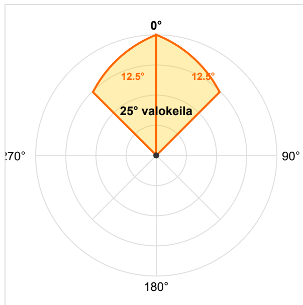
Valonjakokaavio - 25° valokeila kohdevalaisuun
